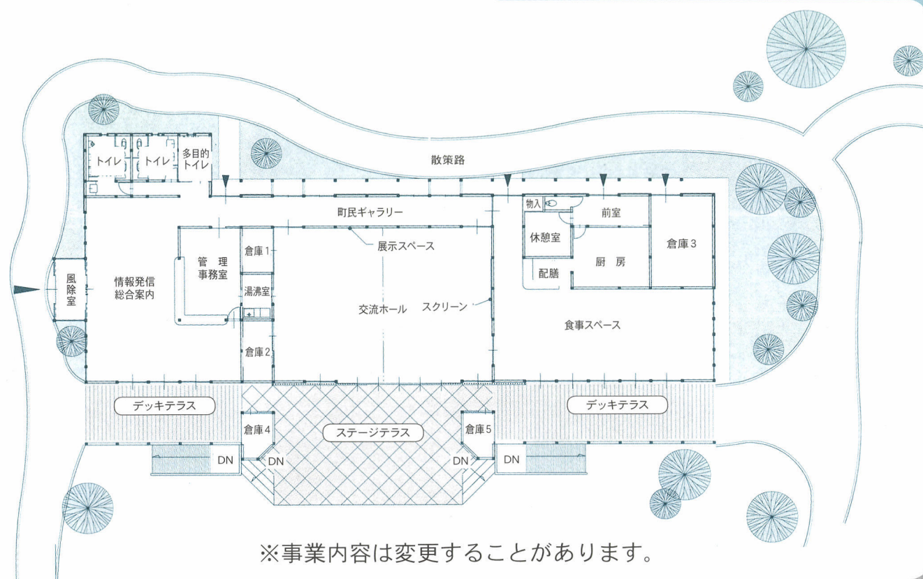
観光交流センター平面図
