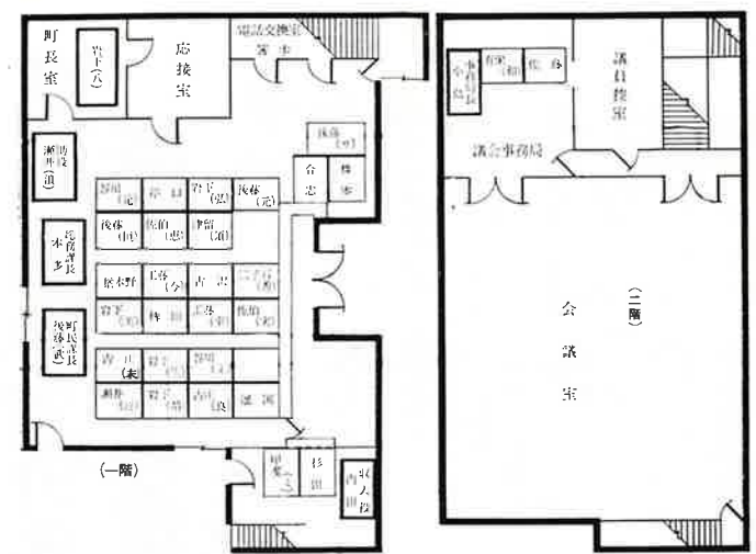
第一庁舎
